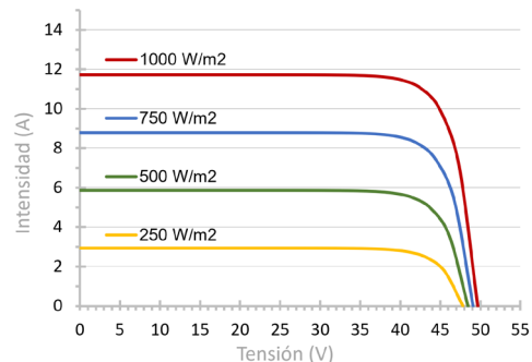
Curvas I-V e Irradiación W/m 2 @ 25°C
